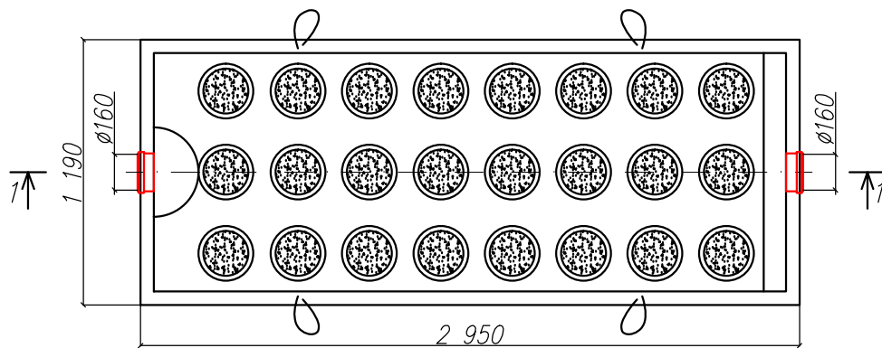
Вид сверху
